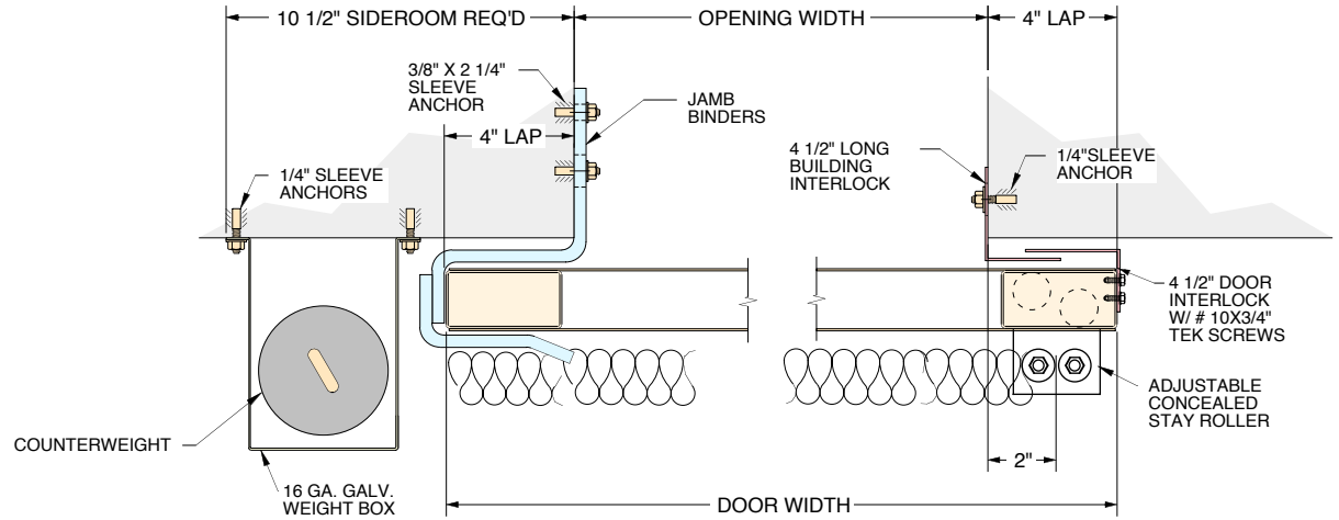
JAMB DETAIL
